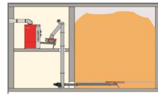
Vertikální spojovací šnek
