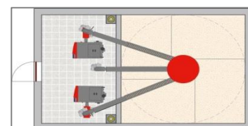
Spojovací šnek pro externí vynašeč
